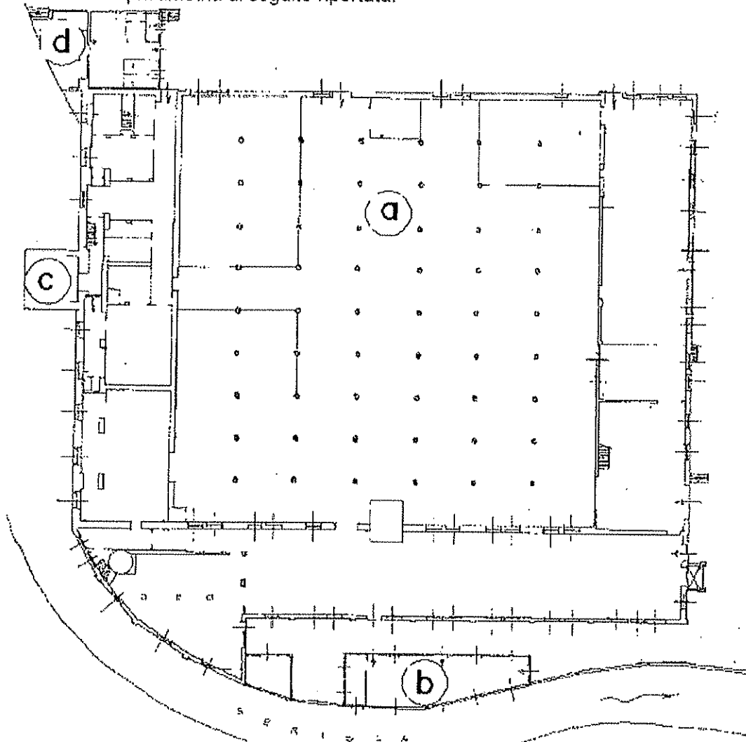
Planimetria piano terra immobile oggetto di perizia
