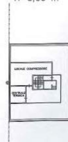
PIANTA PIANO SECONDO H=3,00 m
