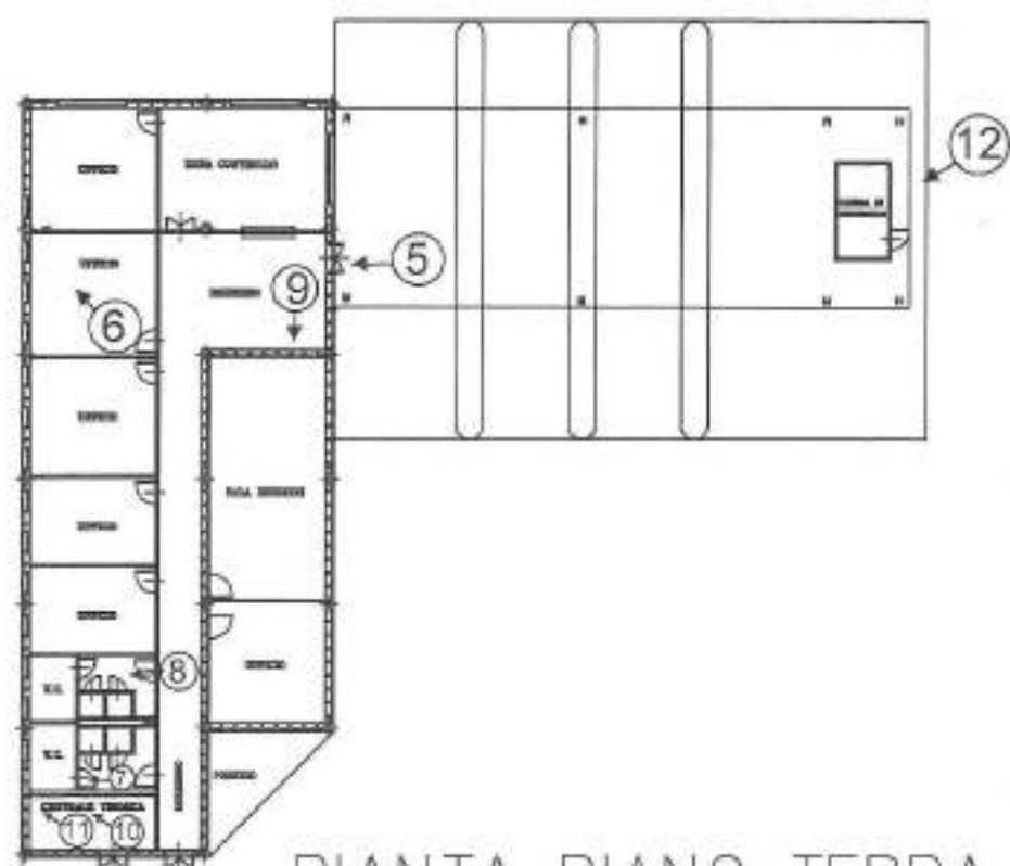
PIANTA PIANO TERRA Cabina Elettrica
