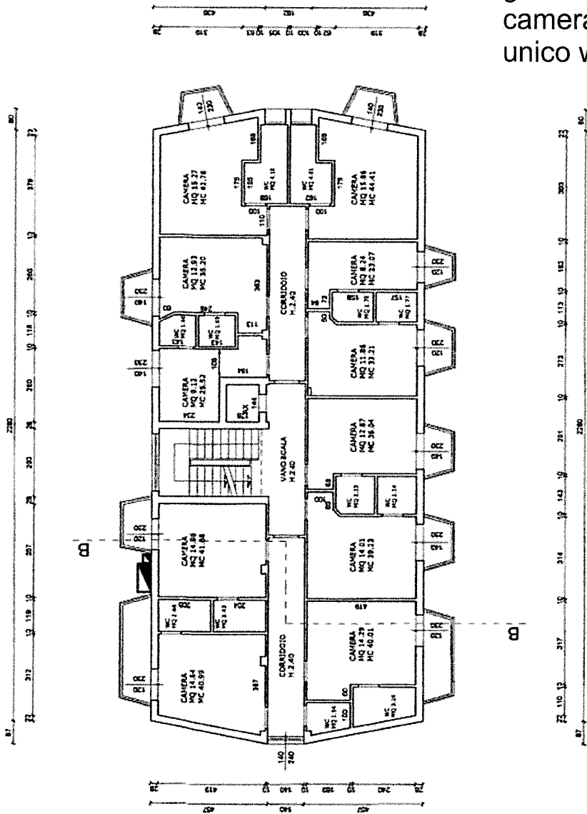
PIANTA PIANO SECONDO N.B. - Aerazione forzata nel w.c. di chi.
