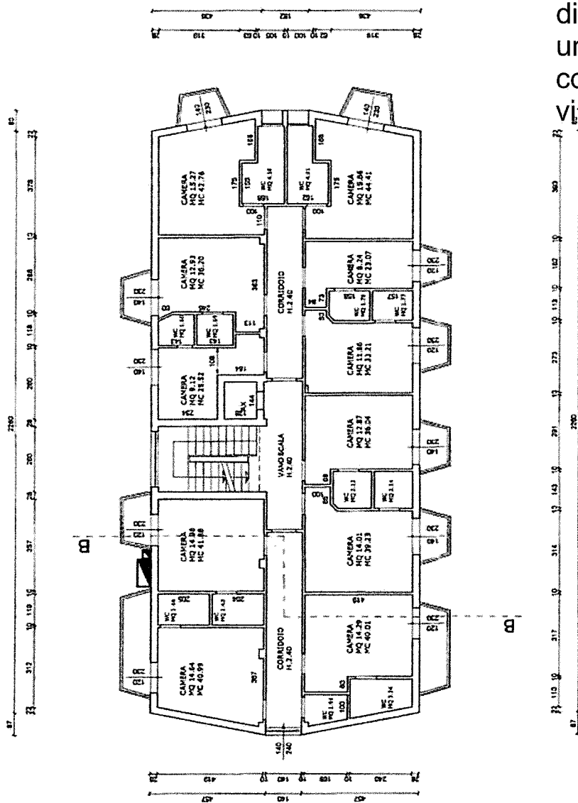
PIANTA PIANO TERZO N.B.: Azione forzata nel w.c. dechi.
