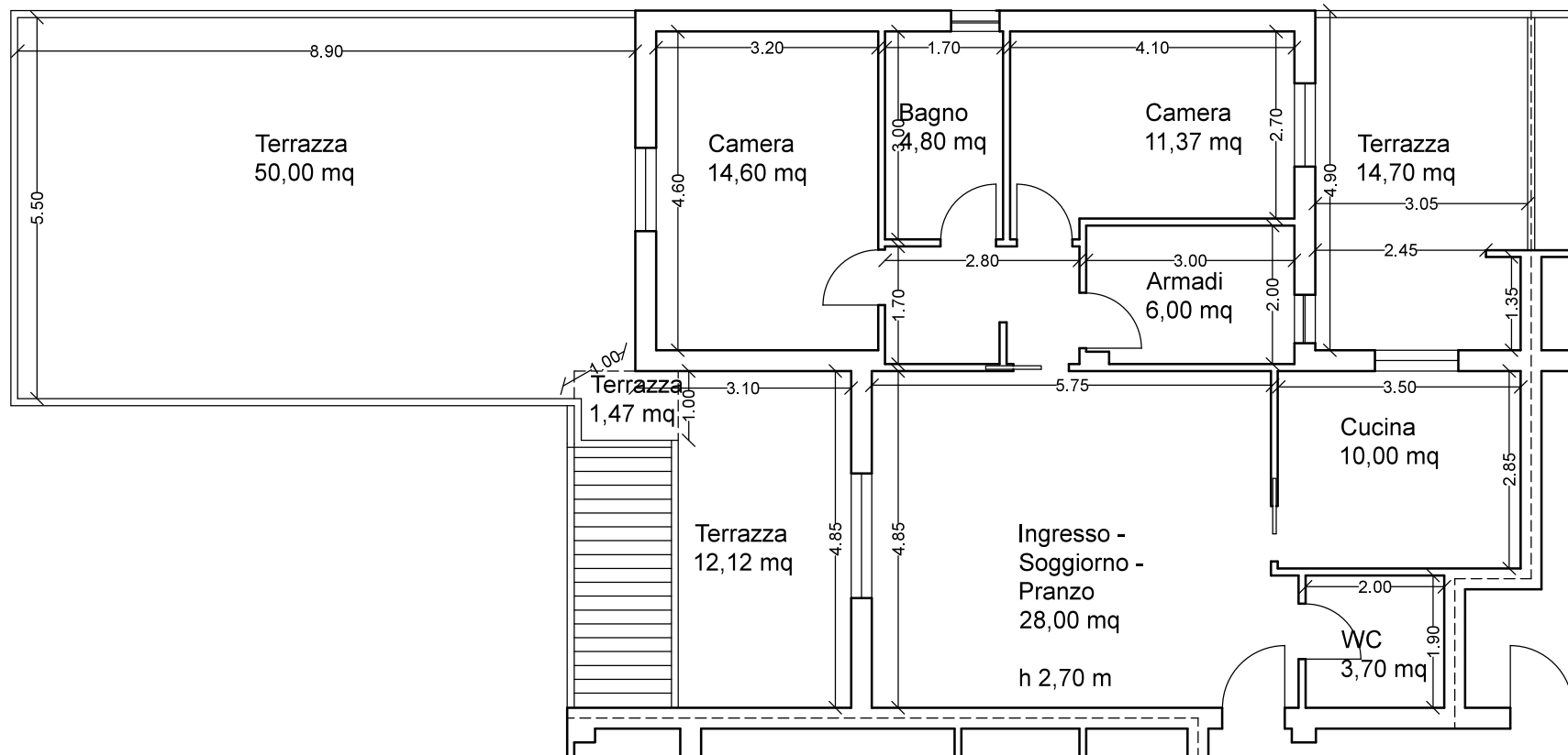
Stato rilevato Piano Terra
