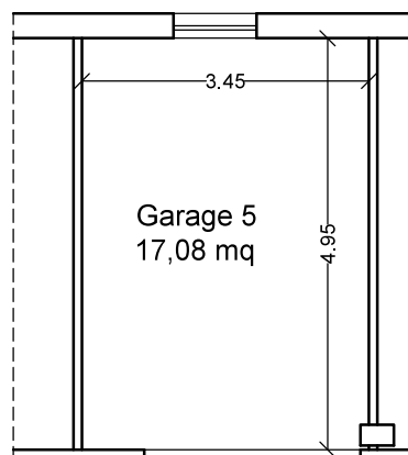
Stato rilevato, licenziato, sovrapposto e accatastato Piano Interrato Garage
