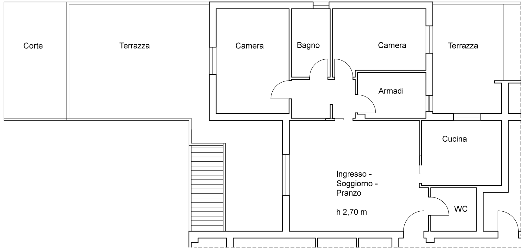
Stato accatastato: Piano Terra
