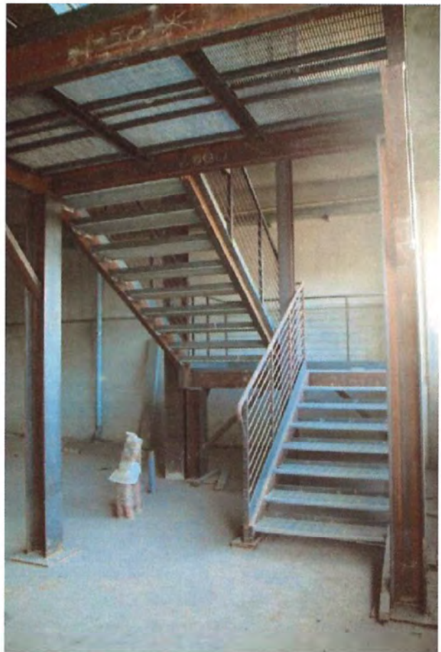
Foto 10. Interno capannone, scala interna
