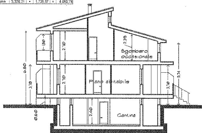
Blocco C SEZIONE TRASVERSALE
